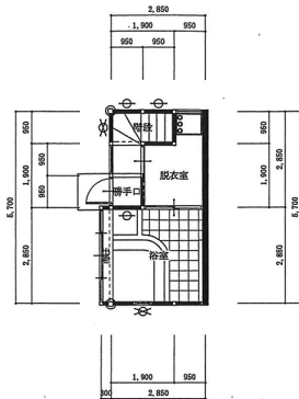
地階平面図 S=1:100
